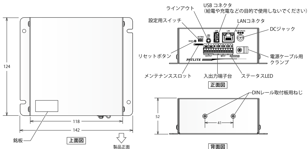
『DRA-2』(株式会社タカチ電機工業製)を使用することで、DINレールへの取り付けが可能。 ※DRA-2はお客様に別途ご用意ください。
