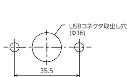
■取付寸法図 (NE-WN-USB)
