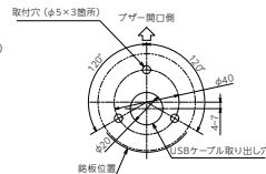
■取付寸法図
